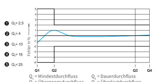
Typische Fehlerkurve
