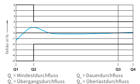
Typische Fehlerkurve
