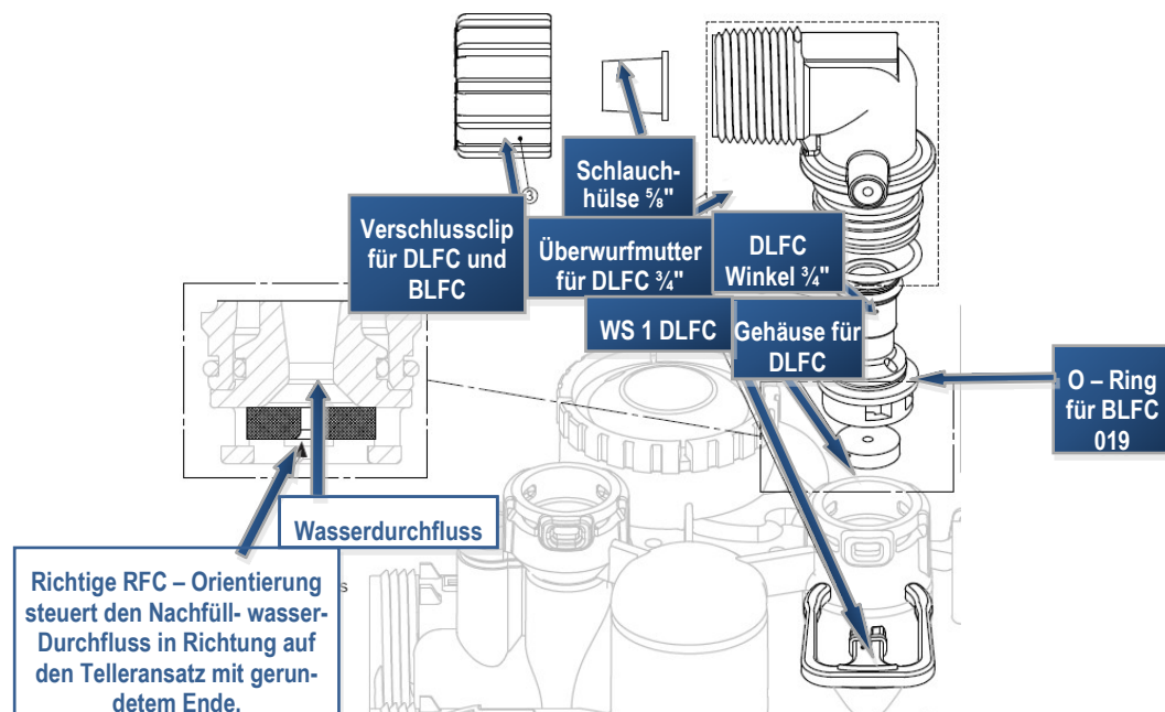
Bild 5. Abwasserblendeneinheit( \frac{3}{4} ").
