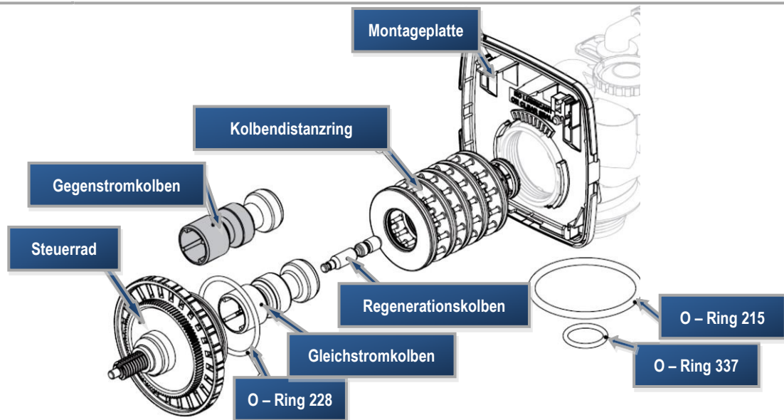
Bild 3. Baugruppe Steuerrad, Gleichstrom- / Gegenstromkolben, Regenerationskolben und Kolbendistanzring.
