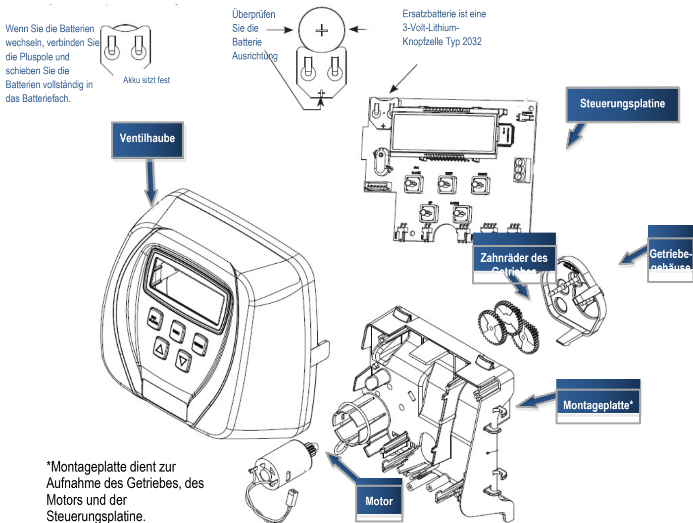
Bild 5. Antriebsbaugruppe.
