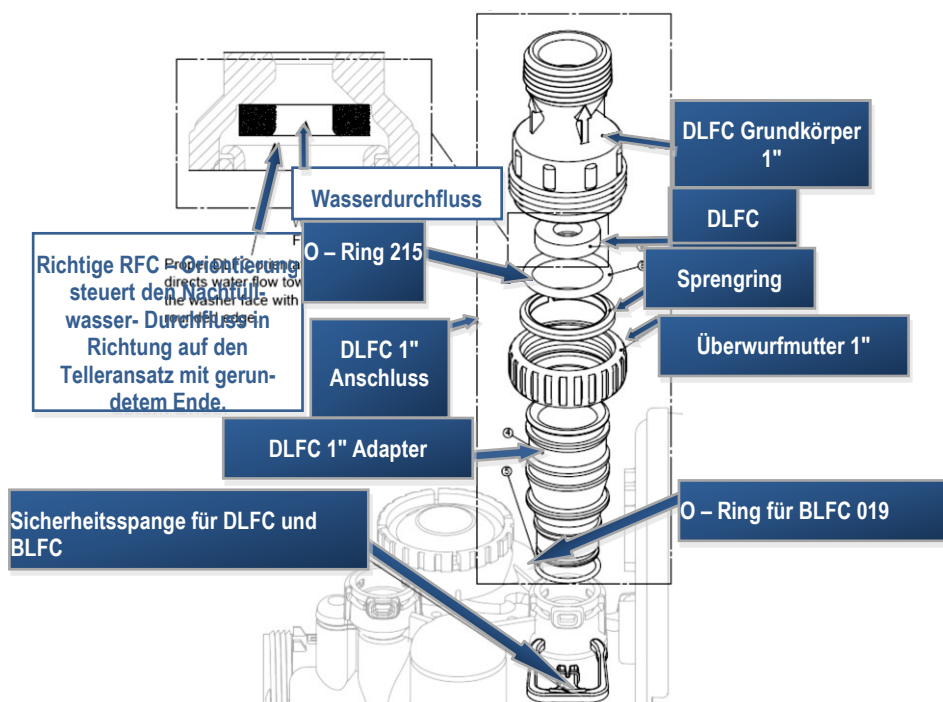
Bild.6. Abwasserblendeeinheit 1".
