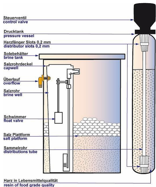
Bild 1. Bestandteile der KadoFilt Kombi CI MONO mit CR 200
