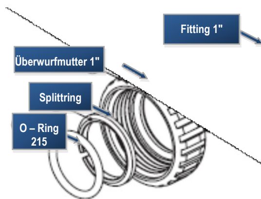
Bild 11. Installationsfittings.
