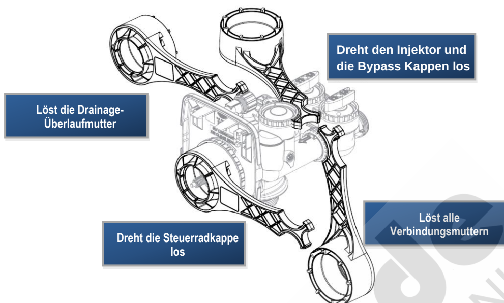
Bild 2. WS1 – Montageschlüssel.
